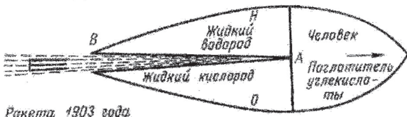
Схема ракеты с прямой дюзой Константина Циолковского
